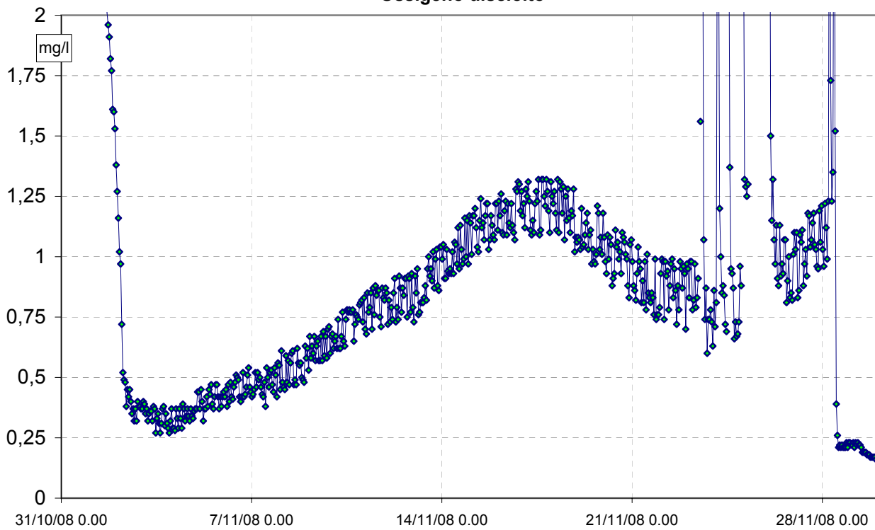
Ossigeno disciolto
