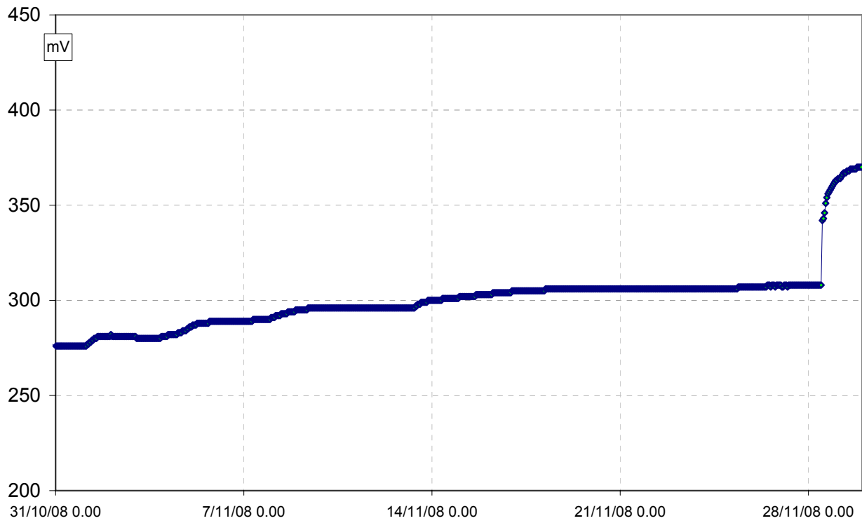
Potenziale RedOx
